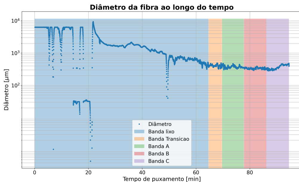
Figura 3: Diâmetro da fibra ao longo do puxamento.
