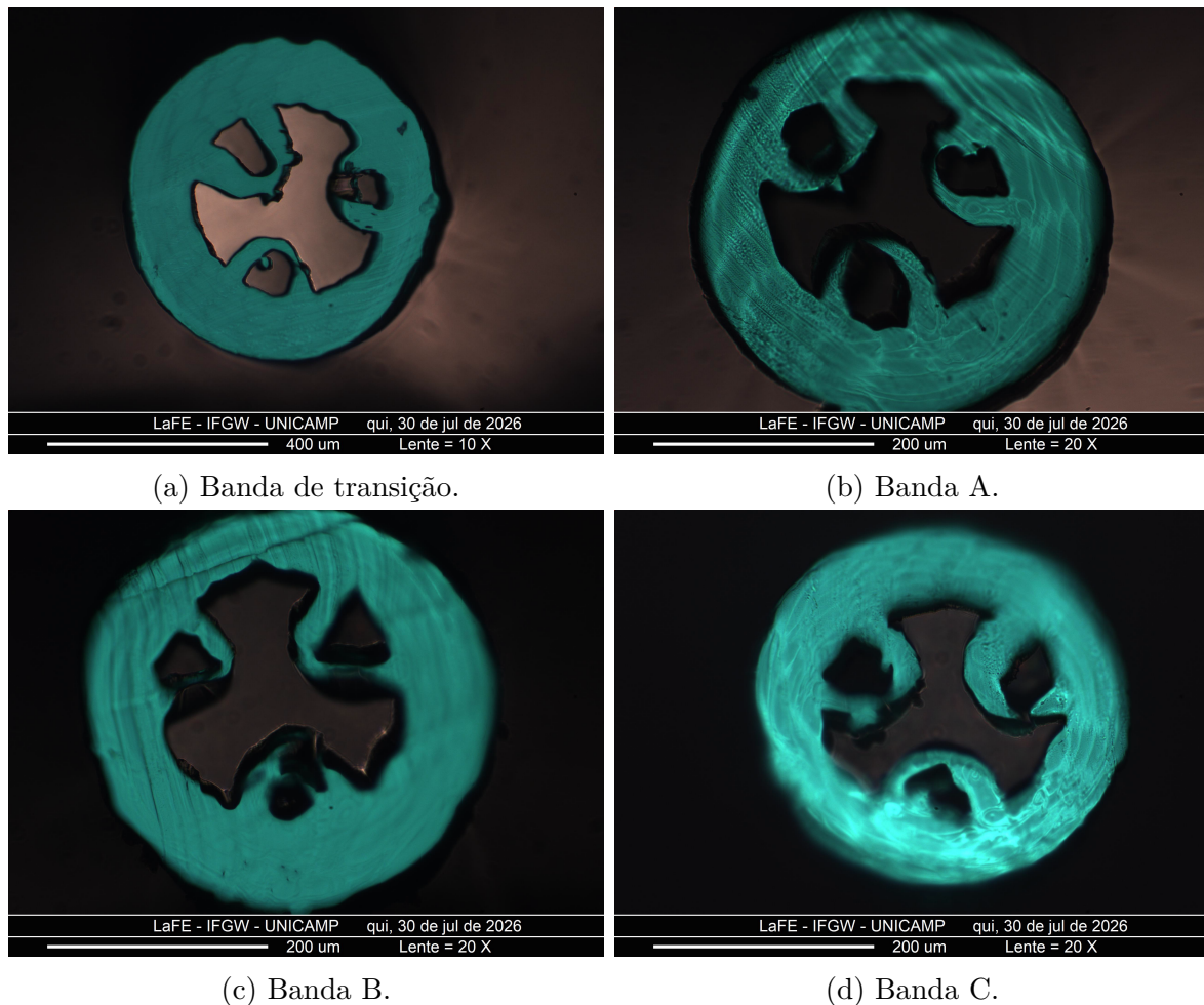
Figura 5: Micrografias do final de cada banda.
