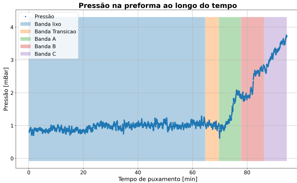
Figura 4: Pressão na preforma ao longo do puxamento.
